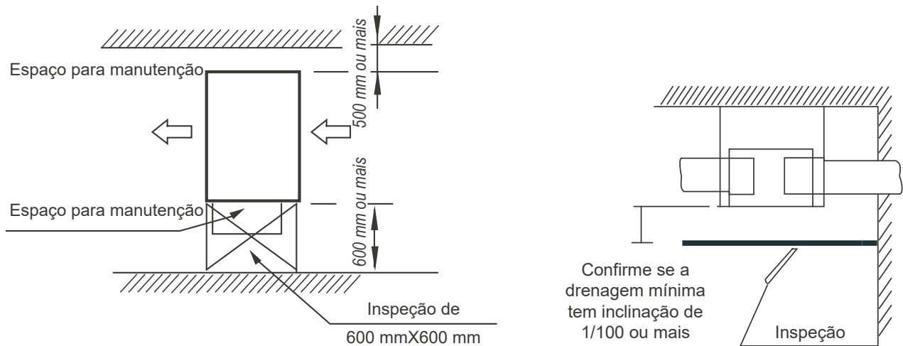
Figura 4: Requisitos de espaço da unidade de renovação de ar (unidade: mm)
