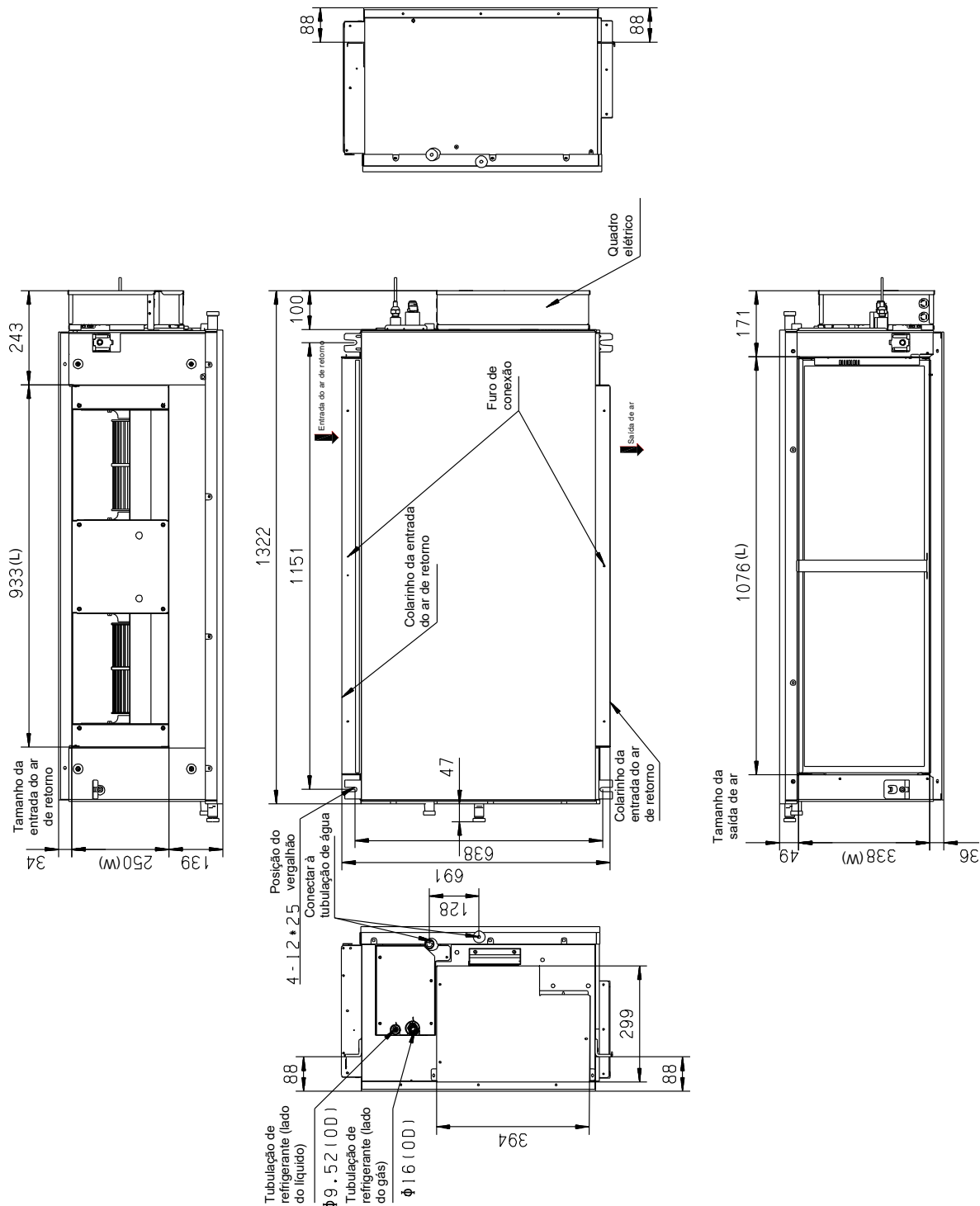
Figura 1: Dimensões do 4TVF0042(48)EF000AA (unidade: mm)
