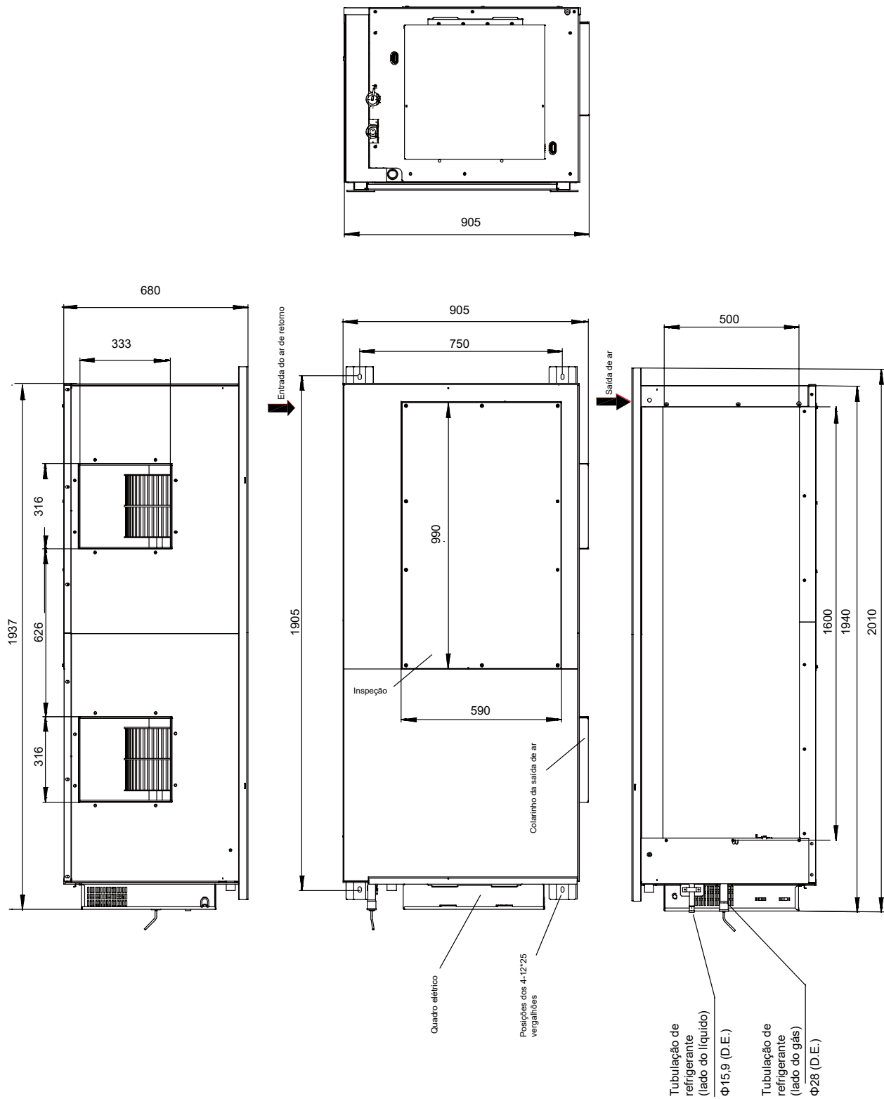
Figura 3: Dimensões do 4TVF0192EF000AA (unidade: mm)
