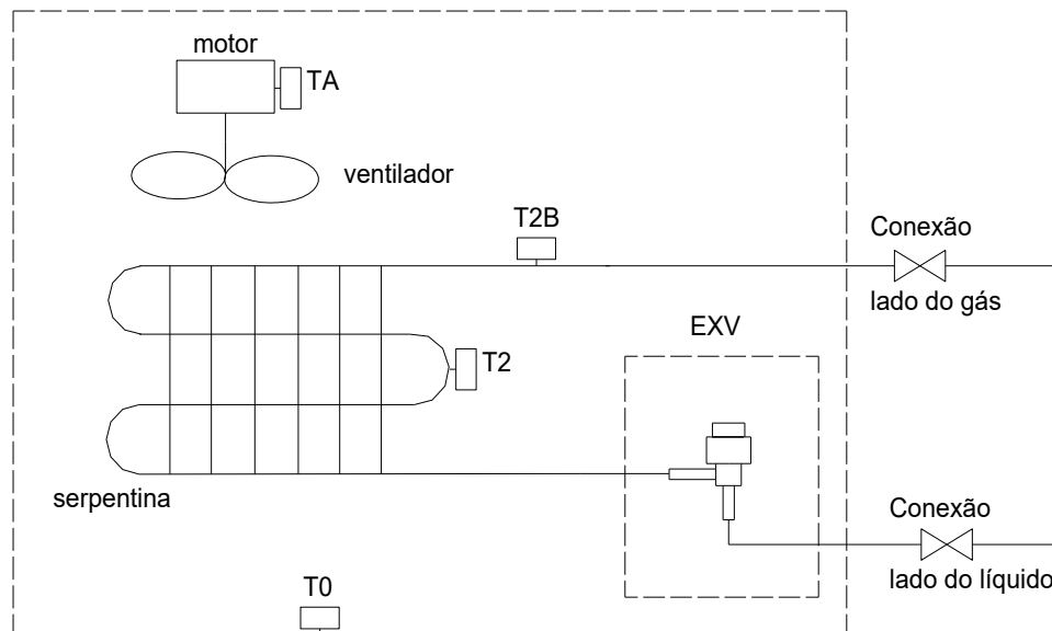
Figura 5: Diagrama de tubulação do 4TVF0042(48-68-85-95)EF000AAFADHN1
