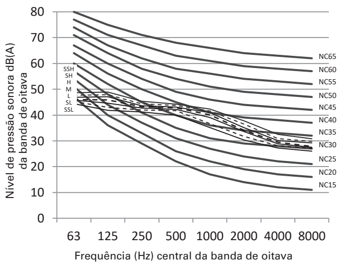
Figura 13: Níveis da banda de oitava do 4TVF0042(48)EF000AA
