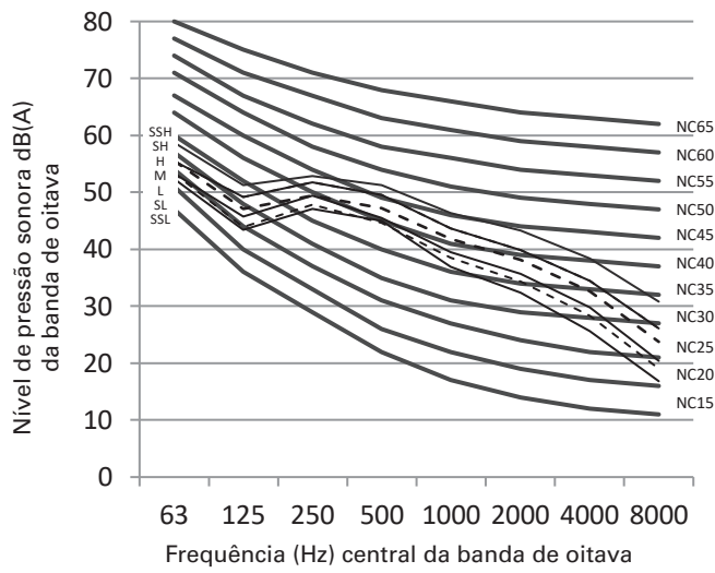
Figura 15: Níveis da banda de oitava do 4TVF0192EF000AA
