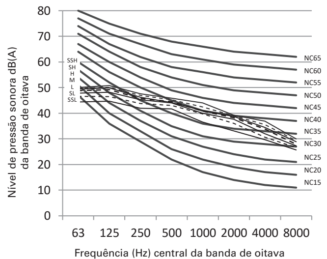
Figura 14: Níveis da banda de oitava do 4TVF0068(85-95)EF000AA
