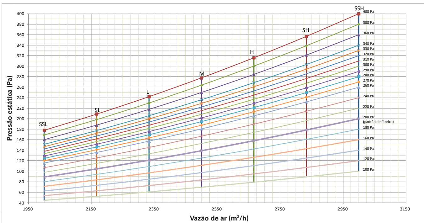
Figura 10: Desempenho do ventilador do 4TVF0068(85-95)EF000AAFADHN1
