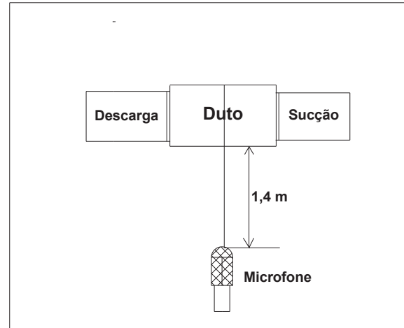
Figura 12: Medição do nível de pressão sonora da unidade de renovação de ar
