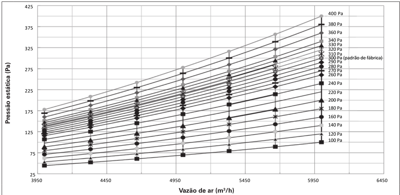
Figura 11: Desempenho do ventilador do 4TVF0192EF000AA
