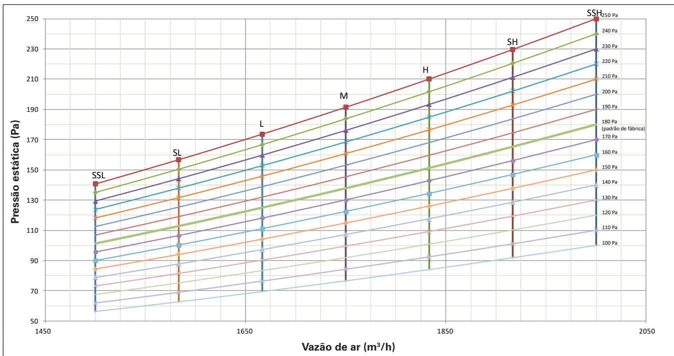
Figura 9: Desempenho do ventilador do 4TVF0042(48)EF000AAFADHN1
